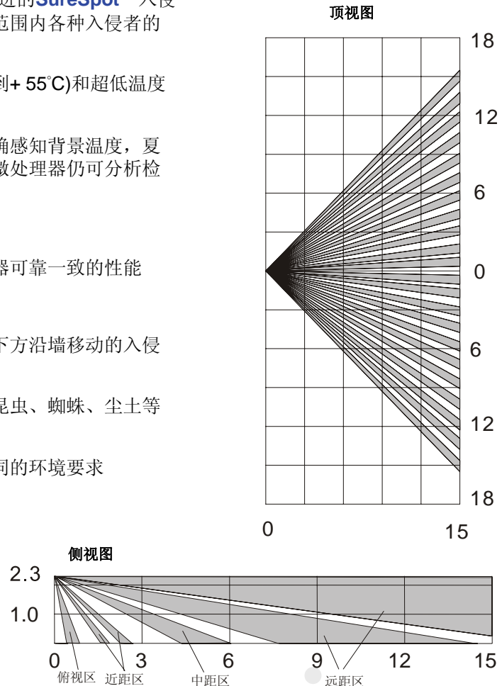
探测器光学视角及保护区示意图
